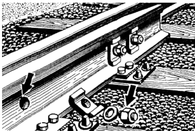
Рисунок 4 – Разрыв контррельсового болта
