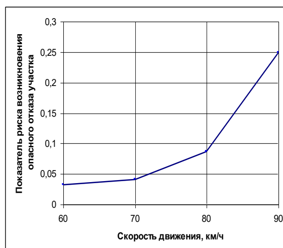
Зависимость показателя риска возникновения опасного отказа участка от скорости движения
