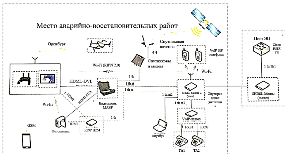
Рисунок 2 – Схема подключения оборудования МКВКС для проведения сеансов ВКС
