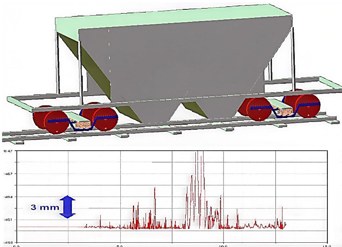
Рисунок 3 – Имитационное моделирование усилий и рисков схода. Вагон-хоппер модель 11-715, тип 930 с тележкой модели 18-100. Обработка в пакете ADAMS/Rail
