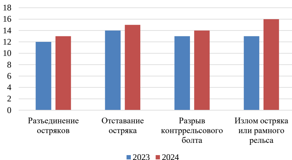
Рисунок 6 – Диаграмма неисправностей стрелочного перевода
