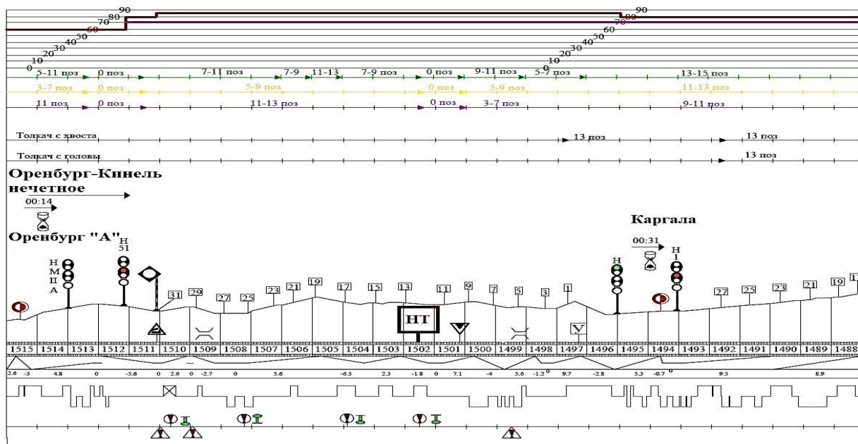
Рисунок 2 – Режимная карта после изменений
