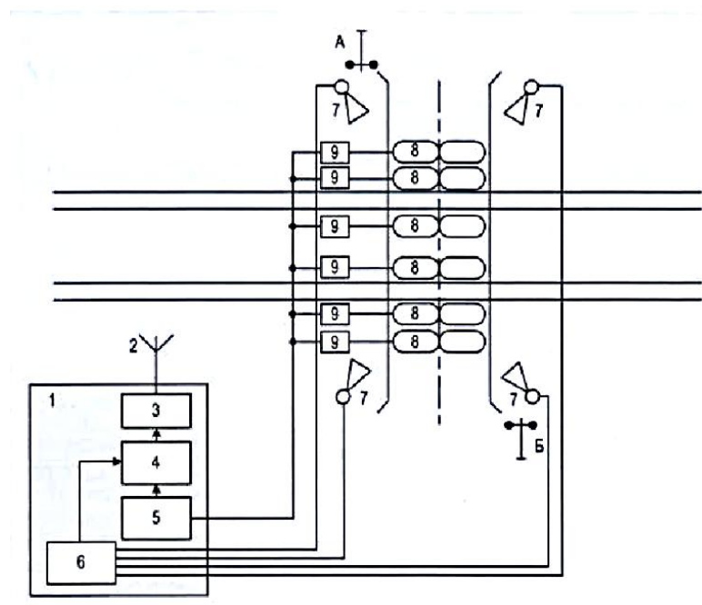
Рисунок 2 – Структурная схема системы контроля и удаленного информирования
