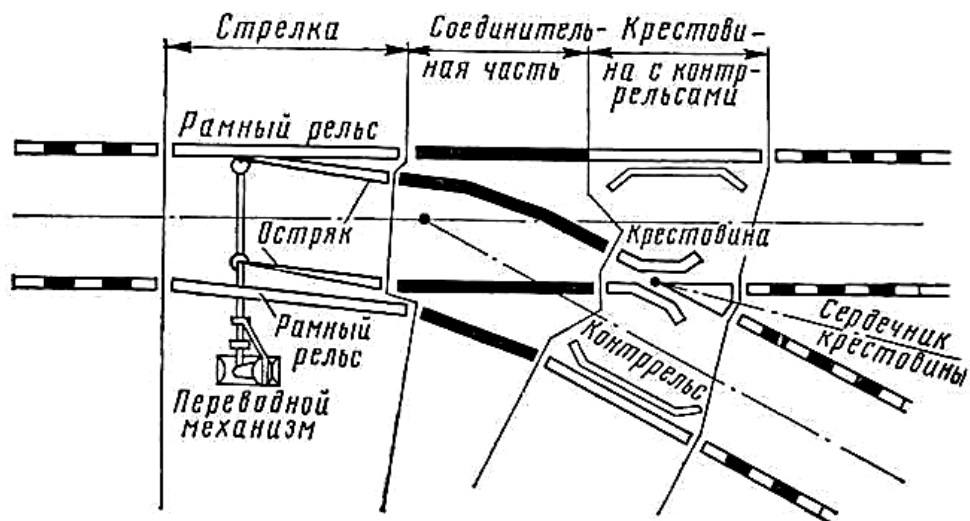
Рисунок 1 – Типовая конструкция стрелочного перевода
