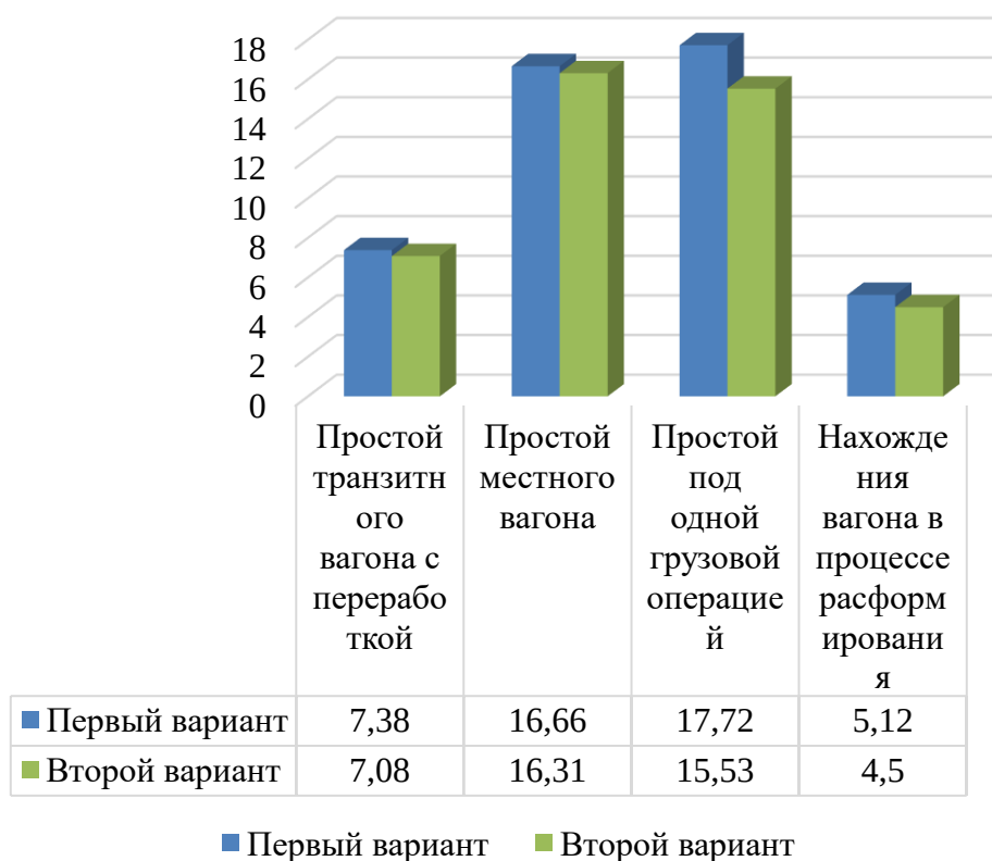
Рисунок 2 – Временные простои до и после удлинения пути (первый и второй вариант)
