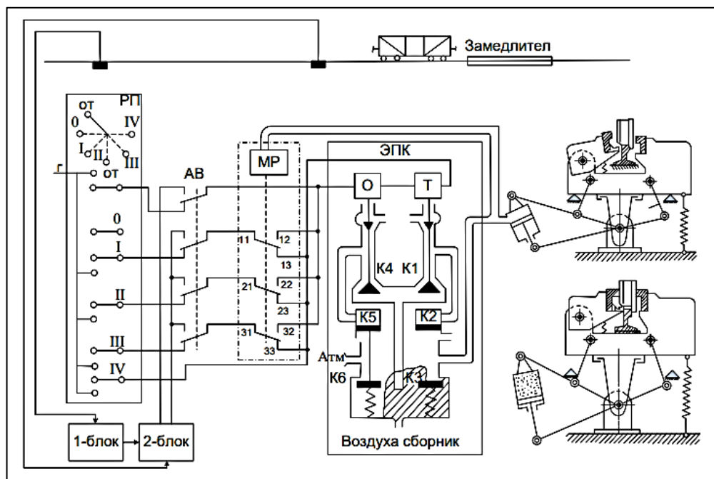
Рисунок 2 – Схема автоматизированной системы роспуска вагонов
