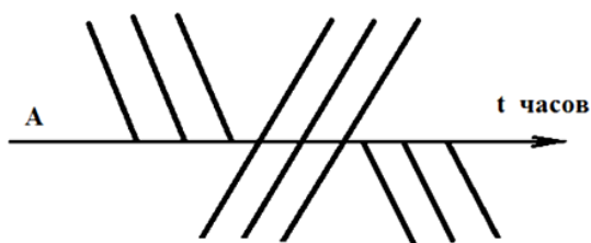
Рисунок 1 – Схема пропуска пакетов поездов при укладке дополнительных путей на разъездах
