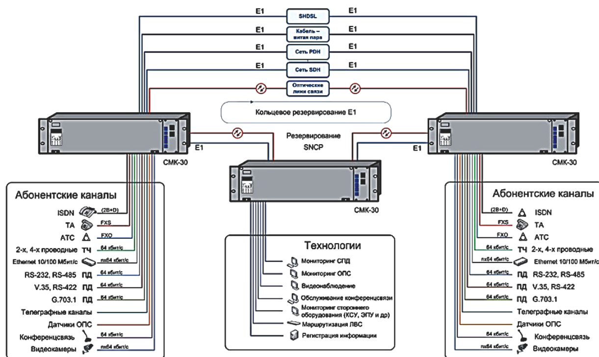
Рисунок 1 – Область применения мультиплексора СМК-30
