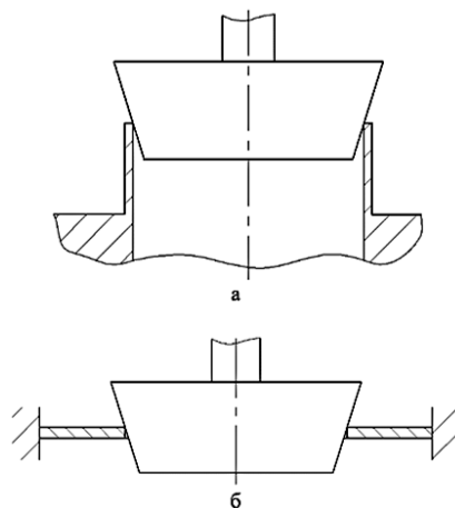
Рисунок 1 – Тонкостенные уплотнения: а – с оболочечным элементом; б – с пластинчатым элементом
