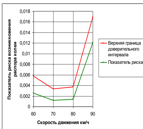
Зависимость показателя риска возникновения распора колес от скорости движения
