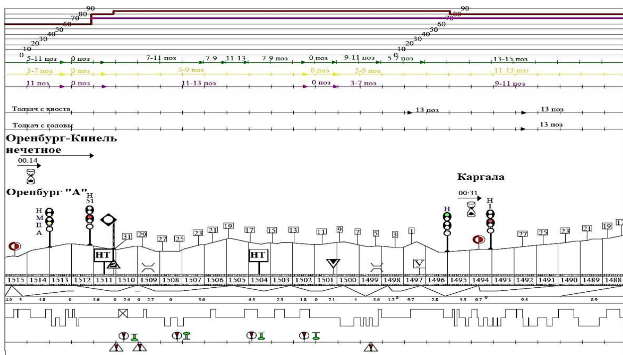
Рисунок 1 – Режимная карта до изменений
