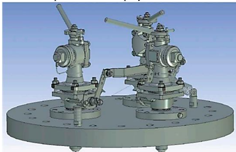
Рисунок 2 – 3D модель ТПА
