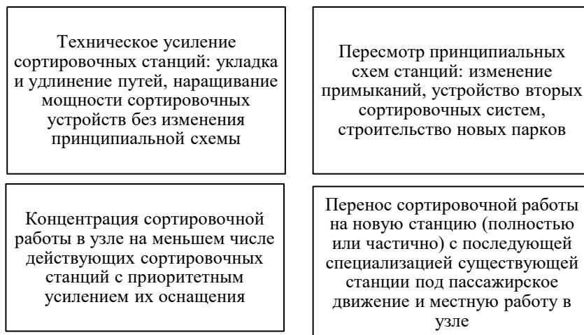
Рисунок 3 – Методы устранения узких мест на железнодорожной станции
