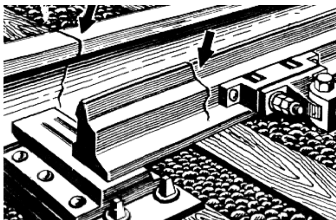
Рисунок 5 – Излом острия или рамного рельса
