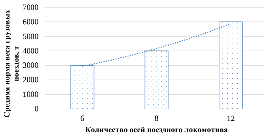
Рисунок 1 – Изменение нормы веса поезда при использовании поездных локомотивов с разным количеством осей
