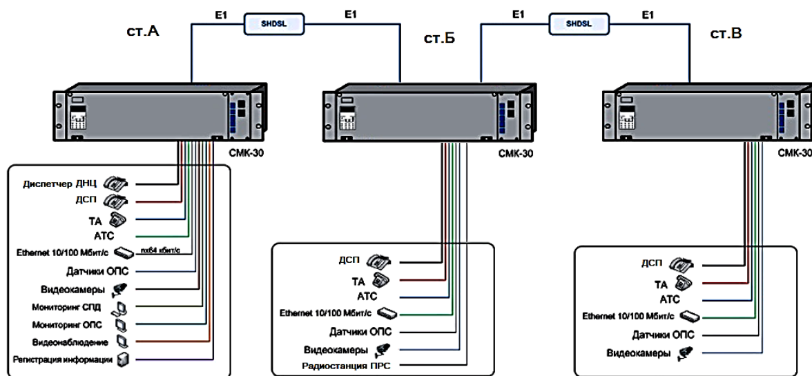
Рисунок 2 – Схема организации ОТС на детской железной дороге на базе мультиплексоров СМК-30
