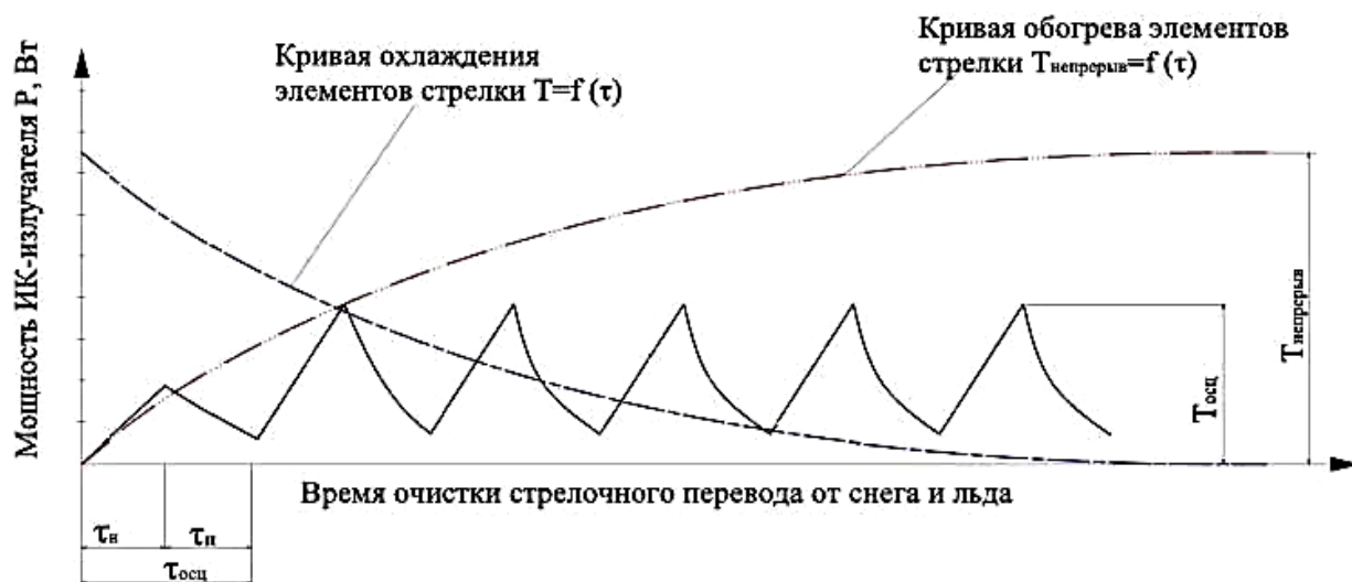
Рисунок 2 – График осциллирующего режима работы ИК излучателя в технологии очистки стрелочного перевода от твердых атмосферных осадков
