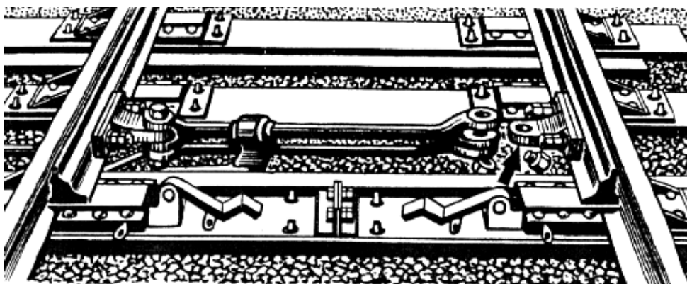
Рисунок 2 – Разъединение остряков
