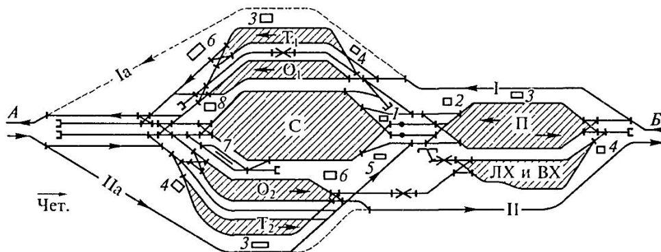
Рисунок 1 – Процесс сортировки вагонов на станции
