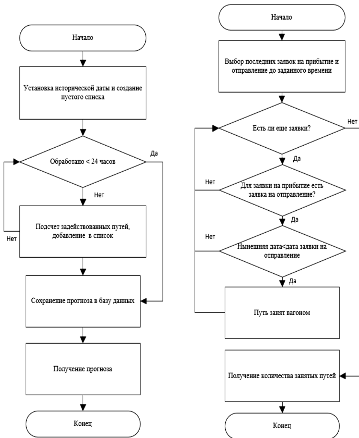
Рисунок 1 – Алгоритмы формирования прогноза и подсчета занятых путей в виде блок-схемы
