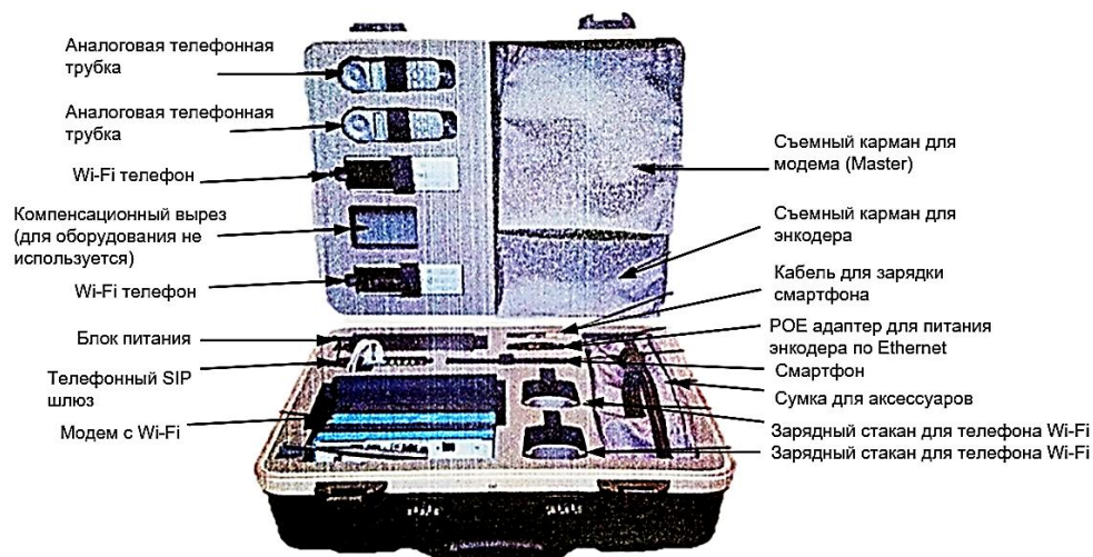
Рисунок 1 – Внешний вид и содержание кейса МКВКС
